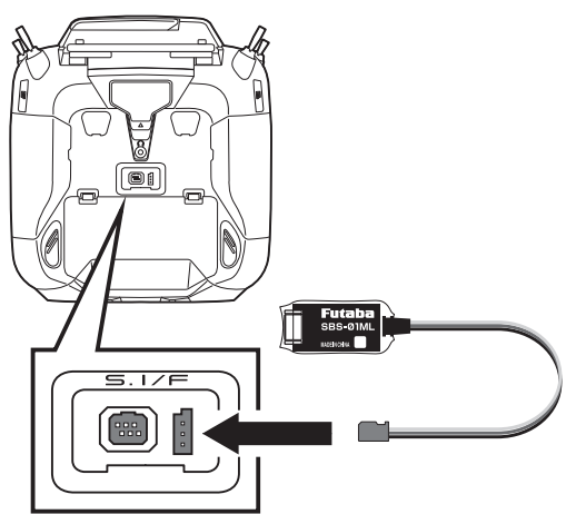
送信機裏面の S.I/F コネクターに SBS-01ML を接続します。
