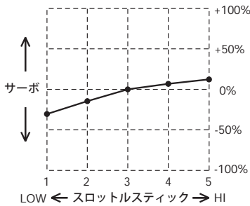
リボリューション NOR 設定例
