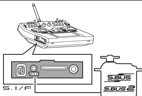
S.BUS/S.BUS2 サーボ
