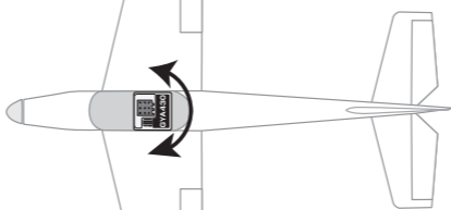
ラダージャイロ搭載位置
