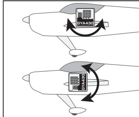
エレベータージャイロ搭載位置
