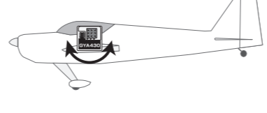
エレベータージャイロ搭載位置
